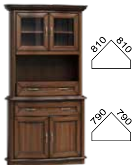
Art. 26 narożny 900 x 1120 x 500
