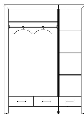
Art. 20 770 x 1500 x 595
